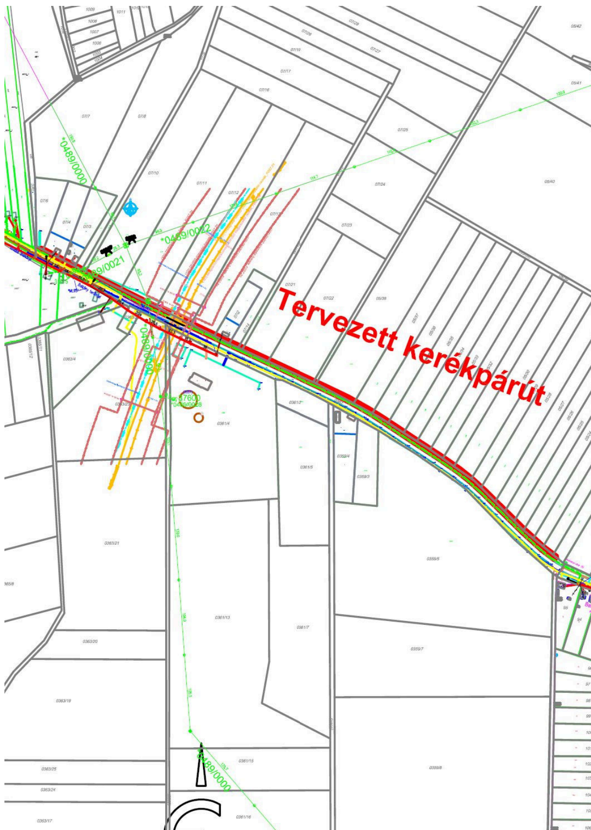
Kerékpárút-építés, átnézeti helyszínrajz (Balkány-Szakoly), forrás úttervező
