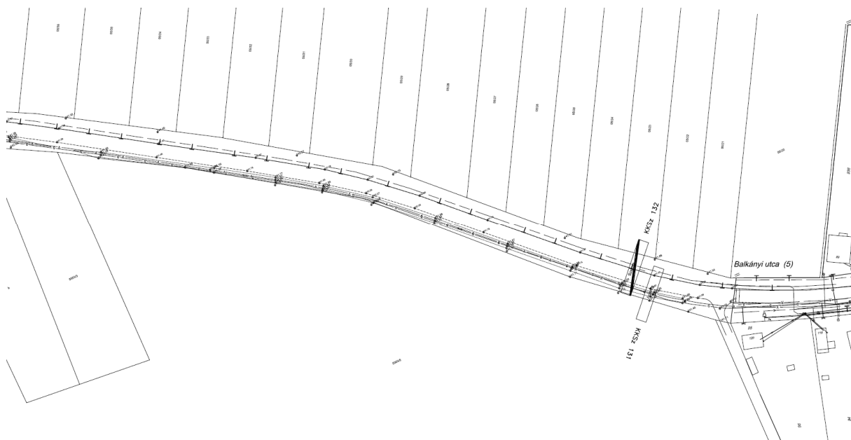
Meglevő állapot helyszínrajz, keleti rész, forrás: úttervező
